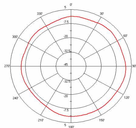
AN2051 E-Plane
