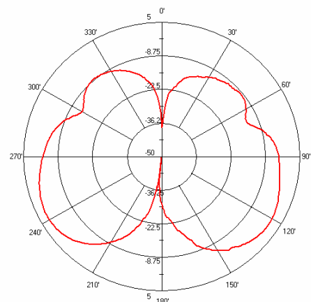
AN2051 E-Plane
